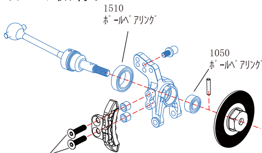
M3x10mm ピン
