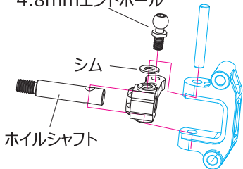
図1 4.8mmエンドボール
