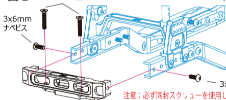
図1 3x20mm 皿ビス
